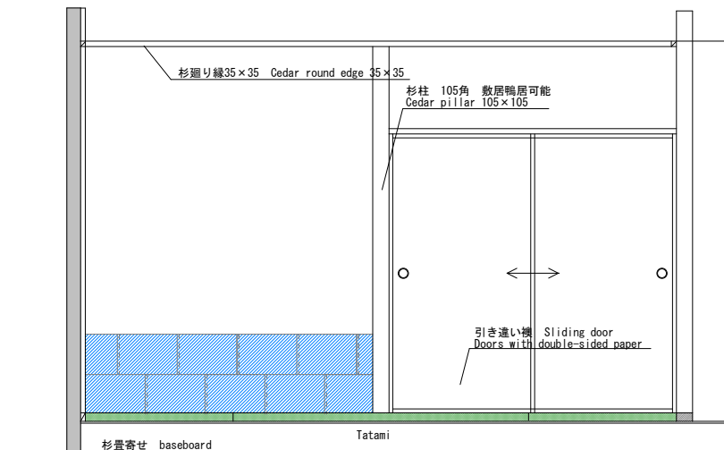
南側展開図 S=1/30 South side elevation diagram
