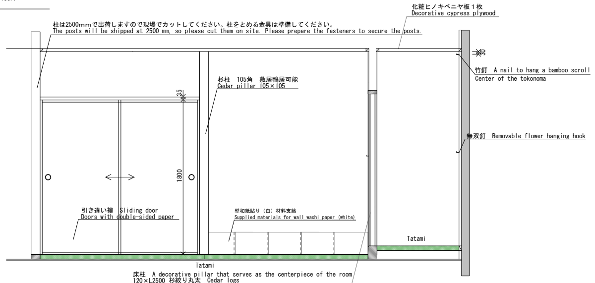
西側展開図 S=1/30 West side elevation diagram
