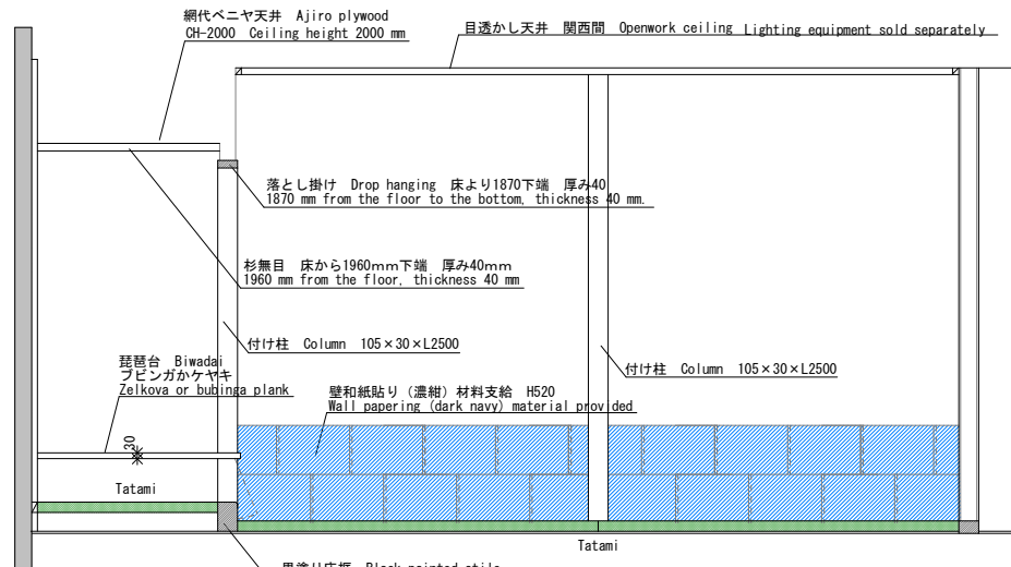
東側展開図 S=1/30 East side elevation diagram
