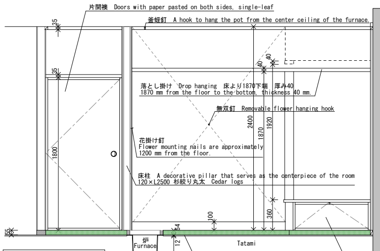
北側展開図 S=1/30 North side elevation diagram
