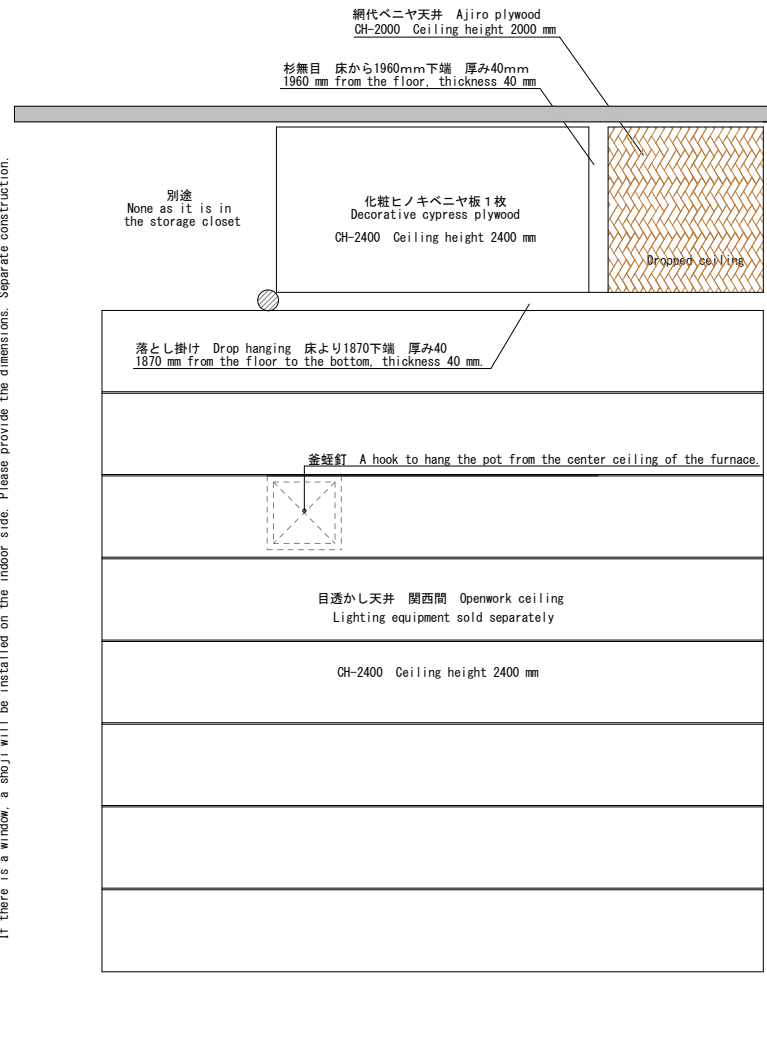
天井伏せ図 Ceiling layout diagram scale1/30
