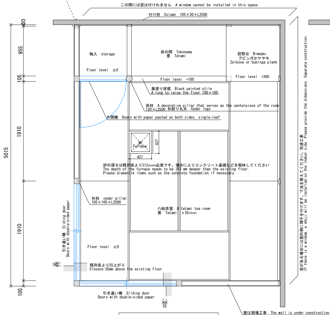
平面図 Floor plan scale1/30
